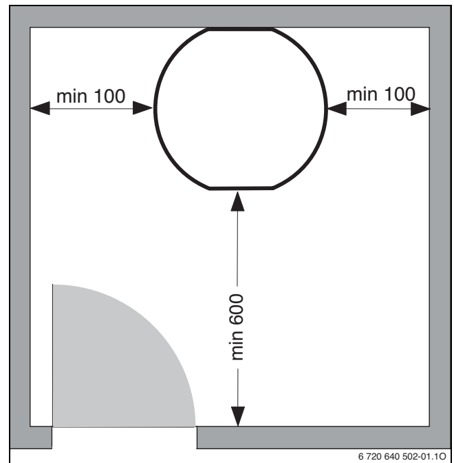
Фиг. 2 Препоръчителни минимални размери на отстояния от стената
