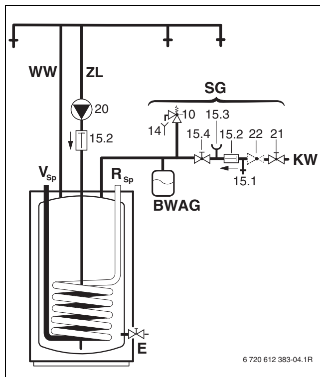
Фиг. 4 Схема за присъединяване от страна на питейната вода
