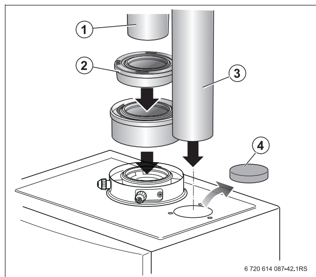
Фиг. 4 Инсталиране на отвеждането посредством отделни тръби
