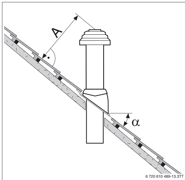
Фиг. 6 Проход на покрив Наклонен покрив
