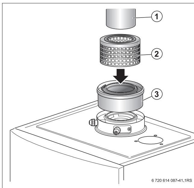
Фиг. 3 Отвеждане посредством единична тръба (зависимо от въздуха в помещението)
