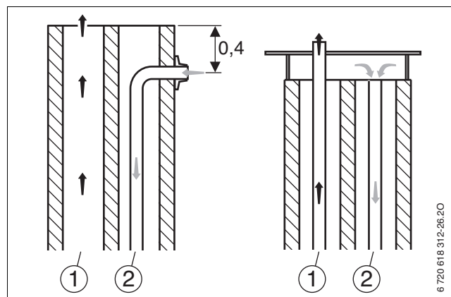
Фиг. 1 Примери за оформление на отвори на устия (размер в m)
