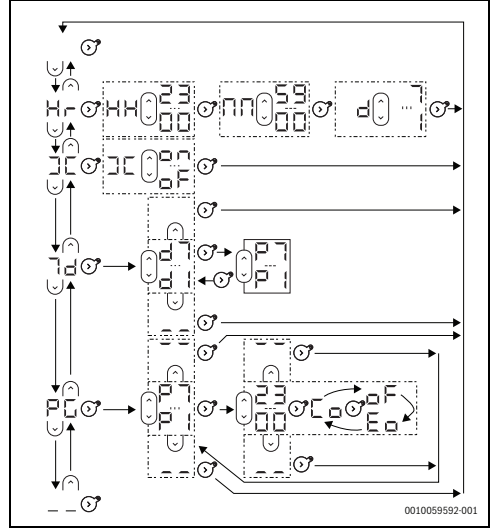
3. ábra Készülék beállítási menü folyamatábrája
