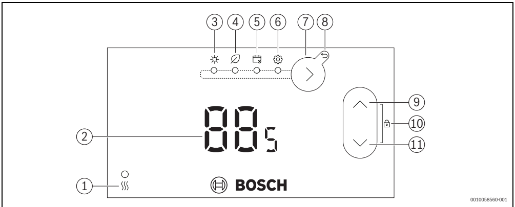
Bild 1 Bedienelemente
