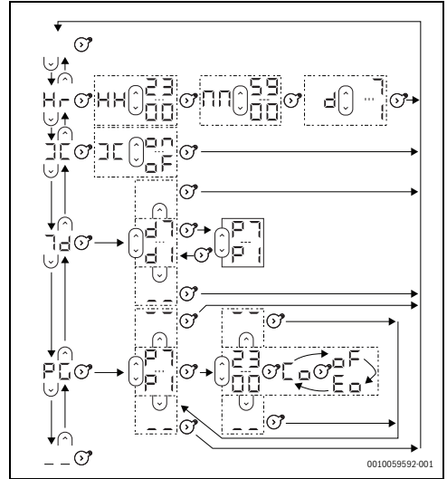
Bild 3 Ablaufdiagramm für das Menü Geräteeinstellungen
