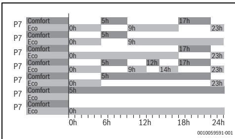
Bild 2 Standardprogramme: P1-P7
