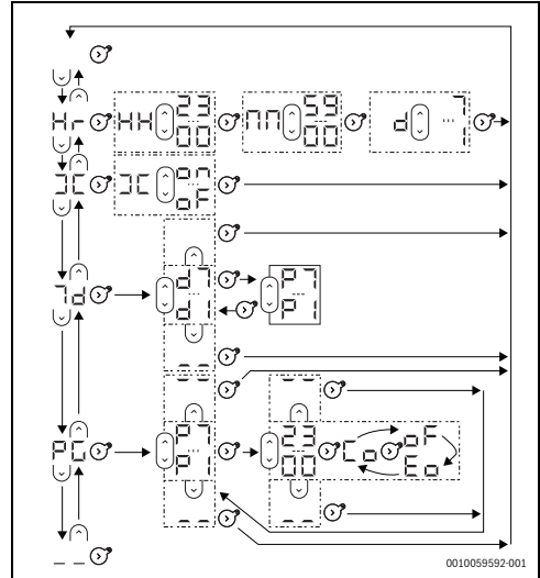
fig. 3 Diagrami i rrjedhës së menysë së cilësimeve të pajisjes
