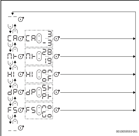
Bild 4 Ablaufdiagramm Expertenmenü
