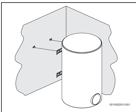
Фиг. 7 Вертикална инсталация (стенен монтаж)
