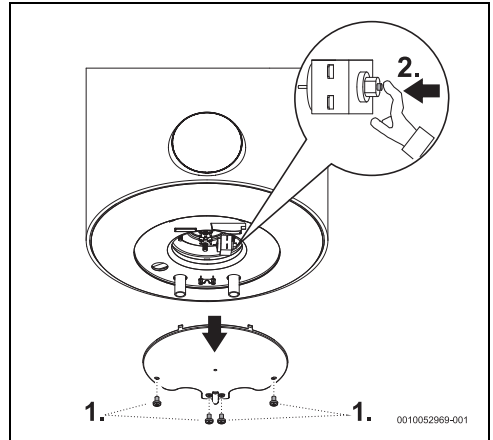
Joon. 10 Ohutustermostaat
