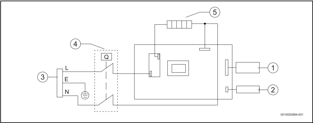
Pav. 11 Jungčių schema
