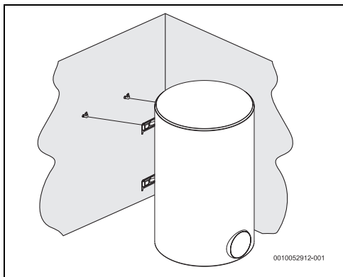
Joon. 7 Vertikaalne paigaldus (seinal kinnitamine)
