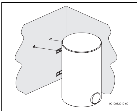
Att. 7 Vertikāla uzstādišana (piemontēšana pie sienas)
