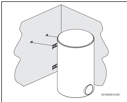
fig. 7 Instalimi vertikal (montimi në mur)
