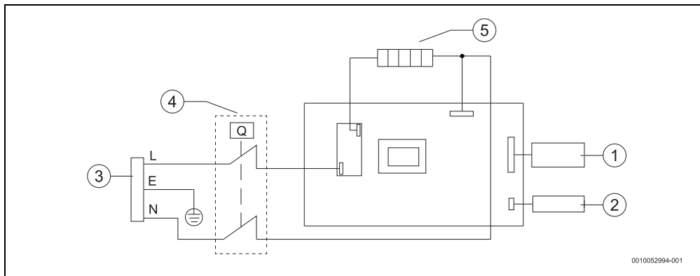
Joon. 11 Ühendusskeem
