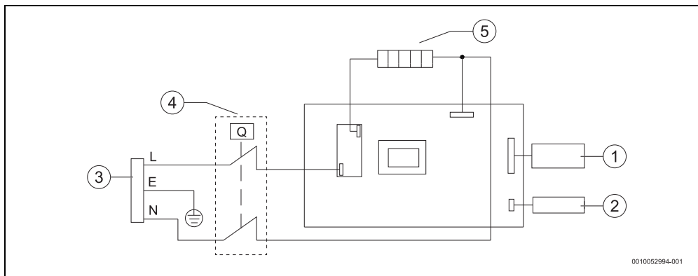
Σχ. 11 Ηλεκτρολογικό σχέδιο σύνδεσης
