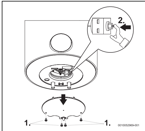
Σχ. 10 Θερμοστάτης ασφαλείας
