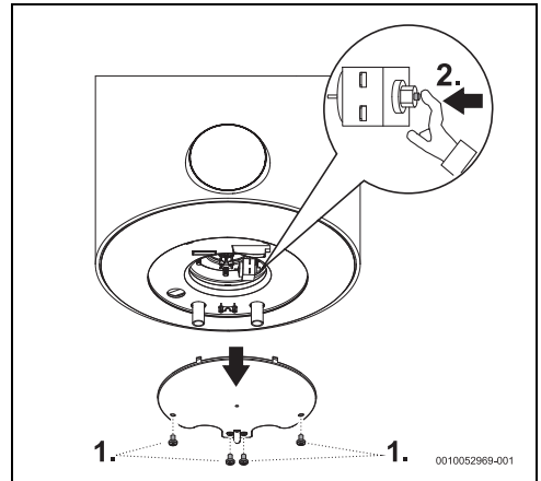
Pav. 10 Apsauginis termostatas
