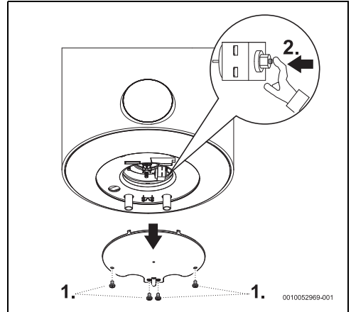
Sl. 10 Sigurnosni termostat
