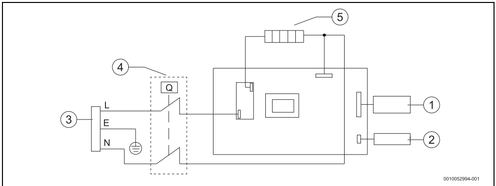
fig. 11 Skema e lidhjeve
