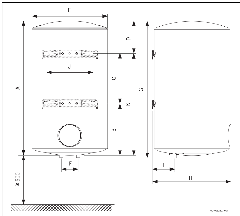
Фиг. 2 Размери в мм (стенен монтаж, вертикална инсталация)
