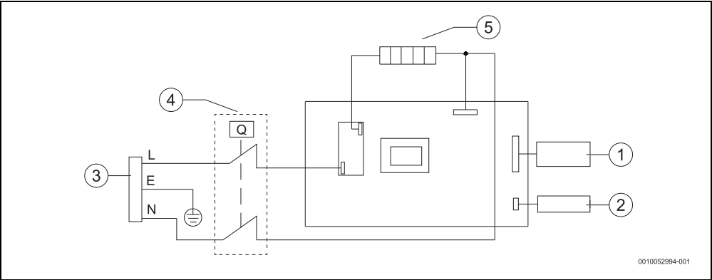
Фиг. 11 Схема на свързване
