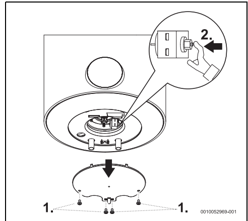
Att. 10 Drošības termostats
