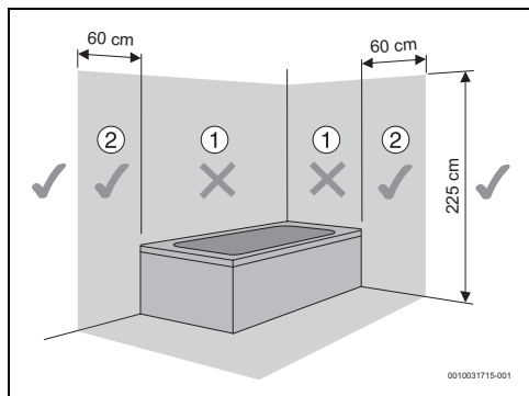
Joon. 5 Kaitsepiirkond
