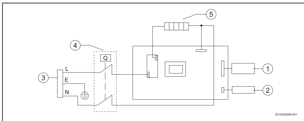
Sl.11 Priključna shema
