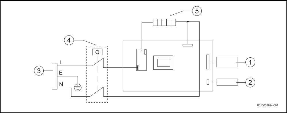
Att. 11 Savienojumu shēma
